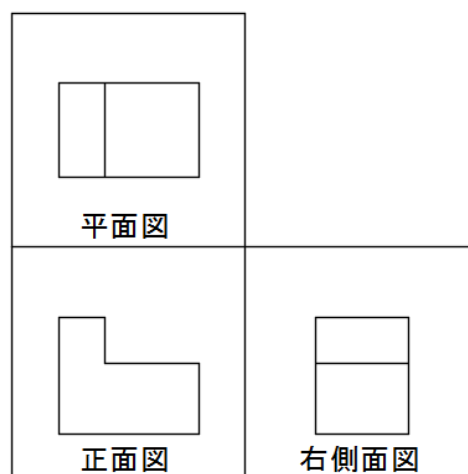
図 3 (b) 第三角法による投影図
