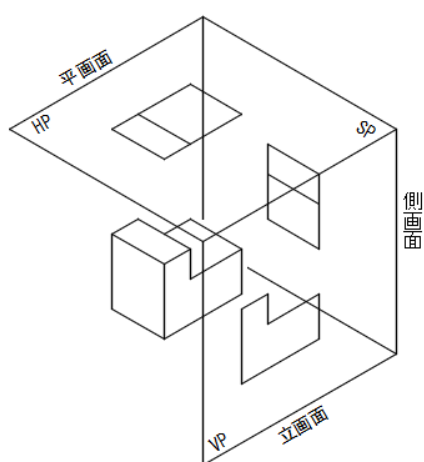
図 3 (a) 第三象限の見取り図
