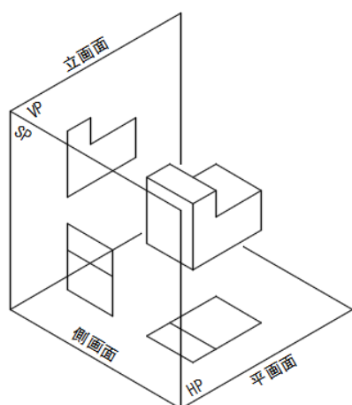
図 4 (a) 第一象限の見取り図
