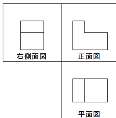
図 4 (b) 第一角法による投影図
