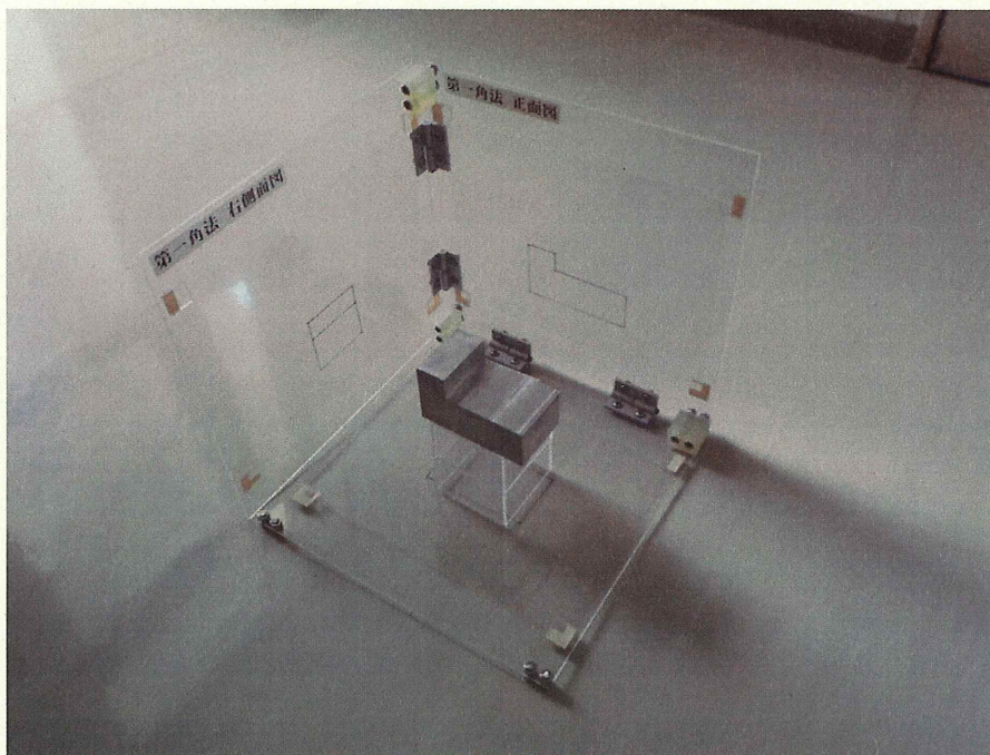
第一角法 模型
