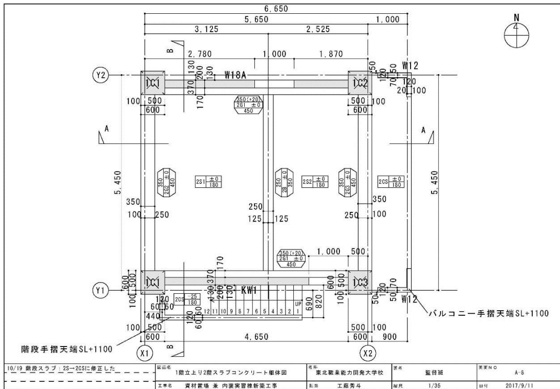
図 3-3 平成 29 年度に施工した 1 階立上り 2 階スラブコンクリート躯体図（平面図）
