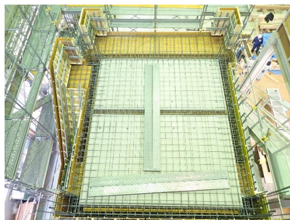
図 3-2-2 平成 30 年度 RC 構造躯体工事 2 階立上り 3 階スラブ施工中
