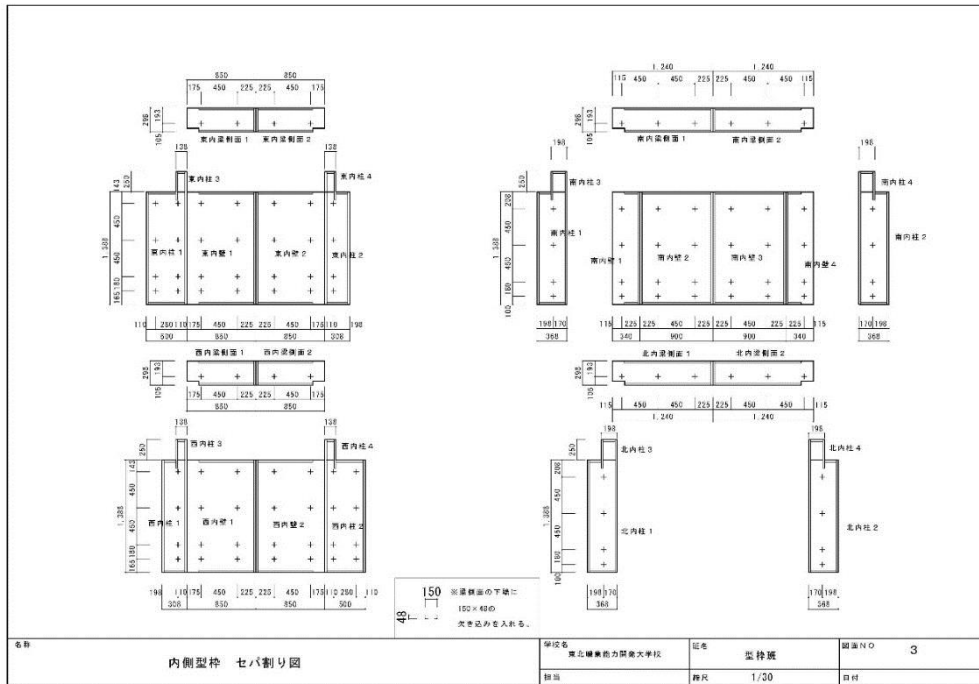
図 3-1-2 標準課題実習（3年）で作成した型枠図面（加工図） 平成 29 年度
