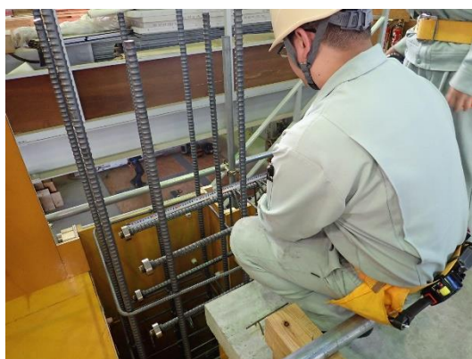
図 3-5-6 梁主筋仕口部での機械式定着
