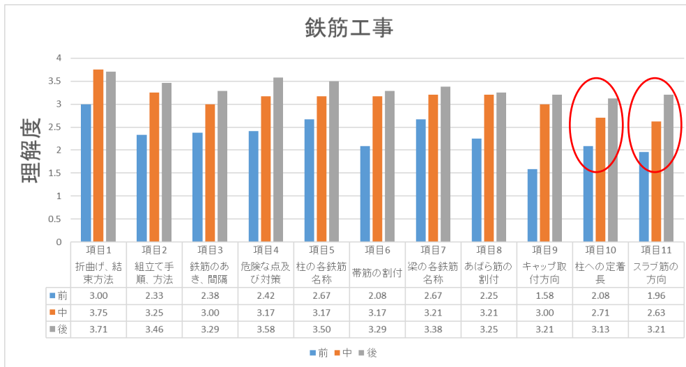
図 4-1-2 鉄筋工事の理解に関するアンケート調査結果
