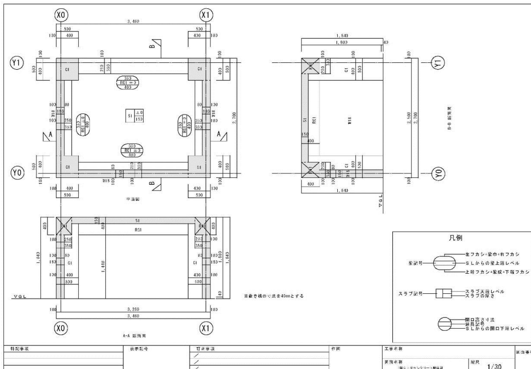
図 3-1-1 標準課題実習（3年）で提示するコンクリート躯体図 平成 29 年度
