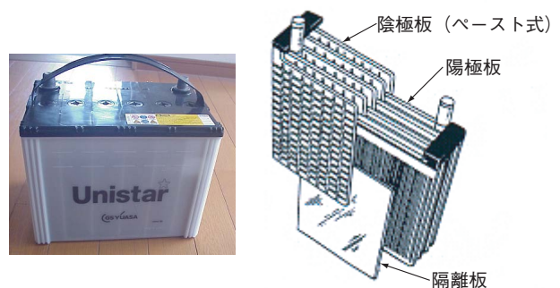
図16 鉛蓄電池とセル略構造図
