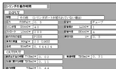
図14 シリンダ動作時間の予測結果
