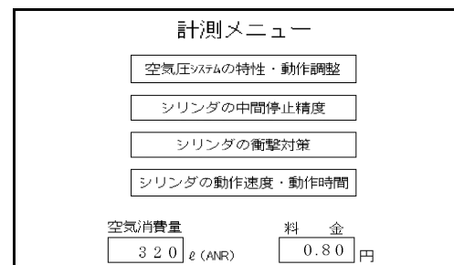
図16 計測結果（エアコスト）
